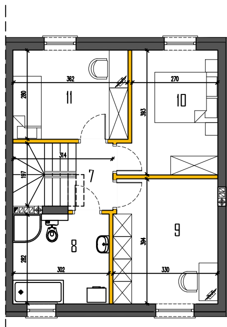
RZUT PIĘTRA
