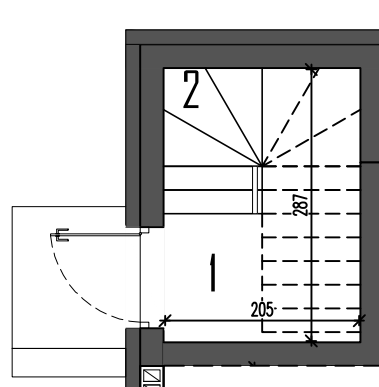
RZUT PARTERU
