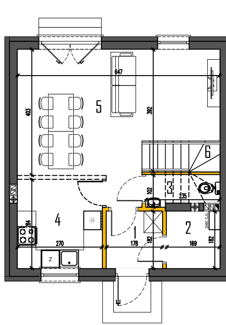
RZUT PARTERU
