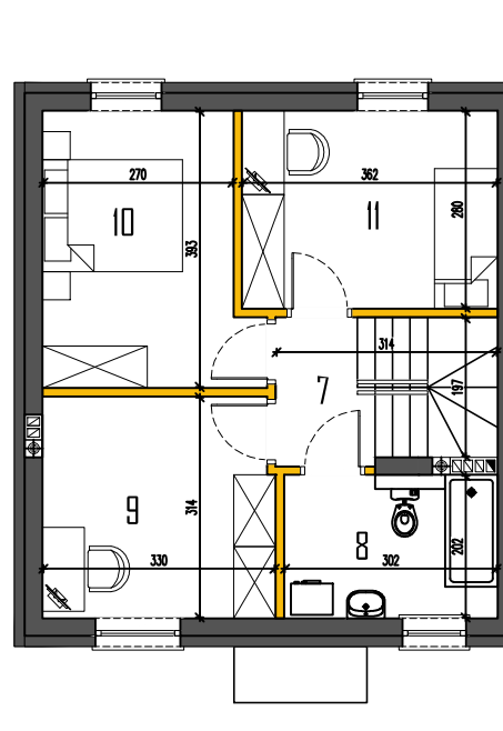
RZUT PIĘTRA
