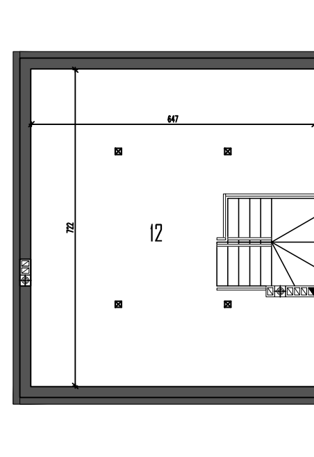
RZUT PODDASZA
