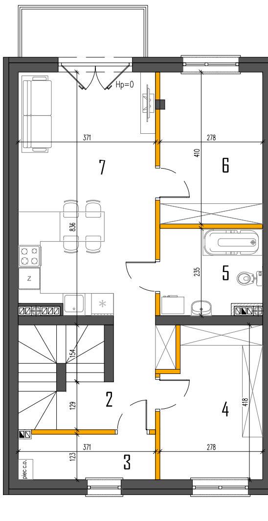
RZUT PIĘTRA
