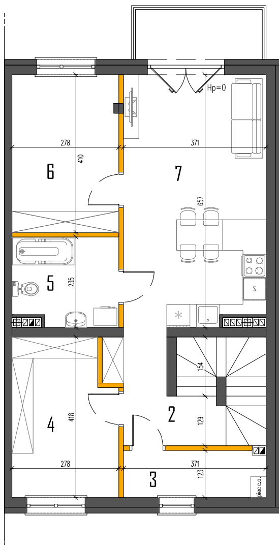
RZUT PIĘTRA
